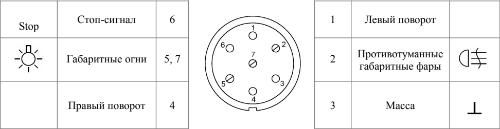
Рис.2. Схема подключения электрооборудования
